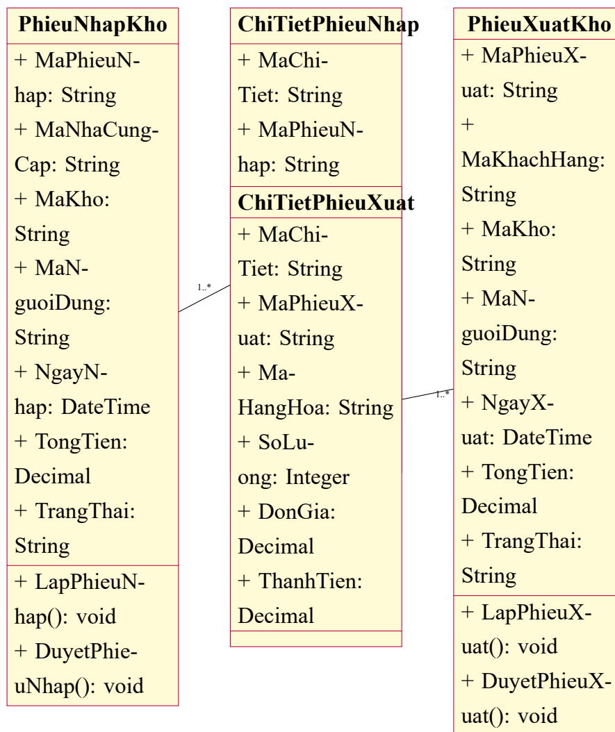
Hình 4.2: Sơ đồ lớp nghiệp vụ nhập xuất kho
