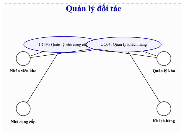
Hình 3.6: Sơ đồ use case phân rã – Quản lý đối tác
