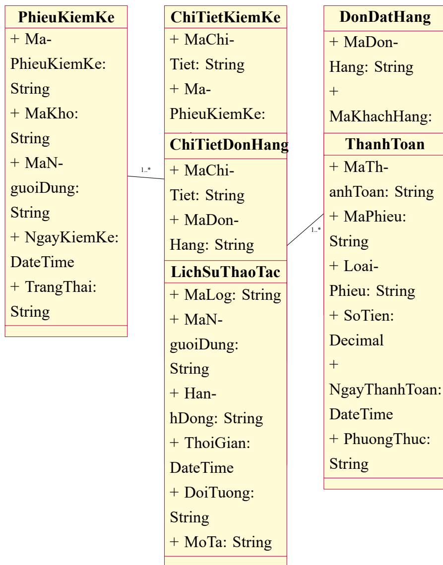
Hình 4.3: Sơ đồ lớp kiểm kê, đơn hàng và thanh toán
